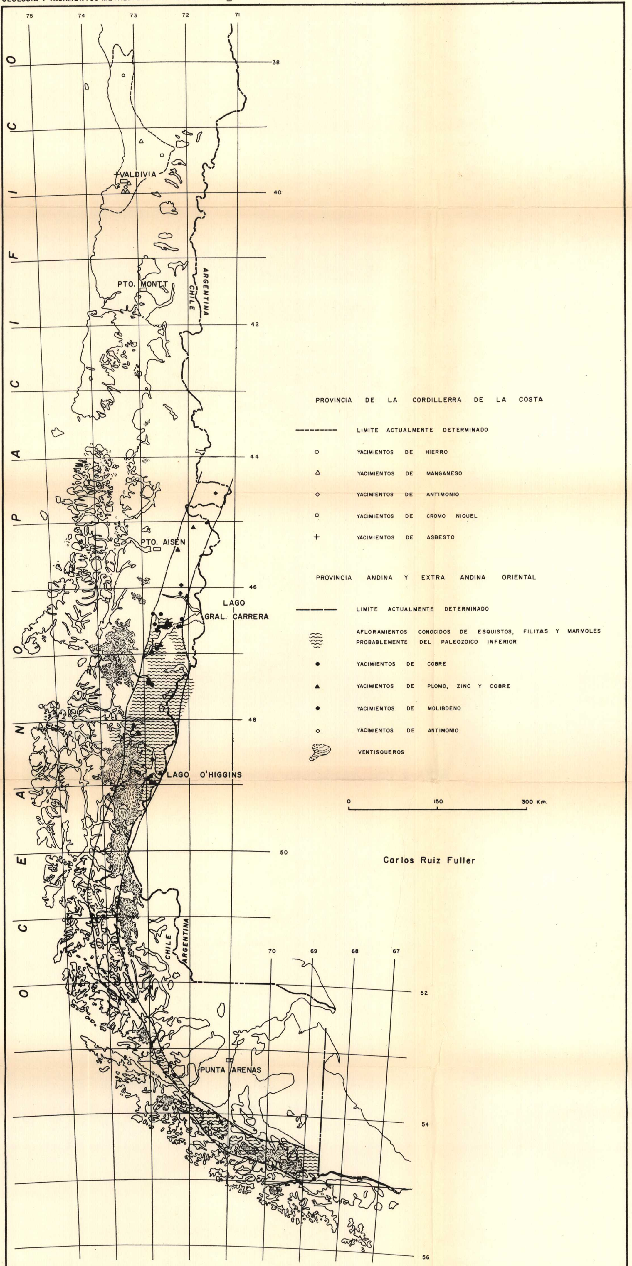
Figura 5.- Provincias Metalogénicas del Sur de Chile.
