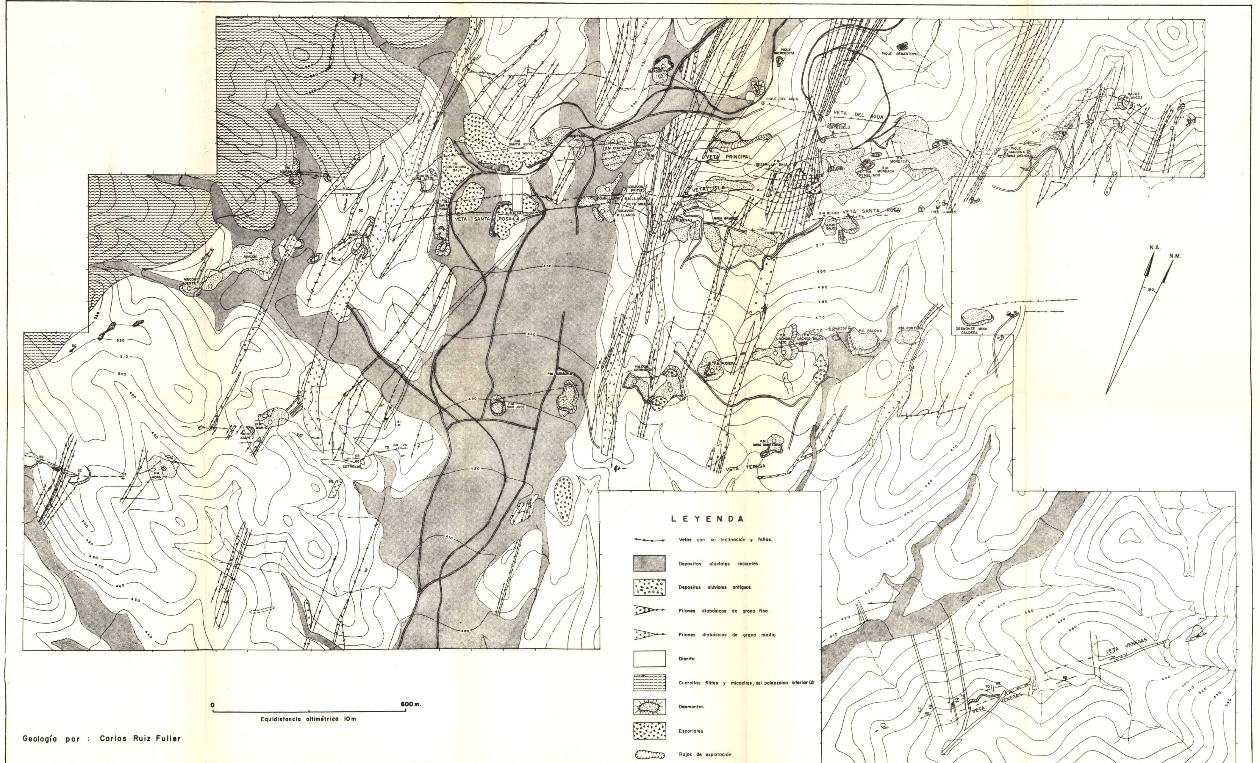
Figura 21.- Mapa geológico del distrito de Carrizal Alto.
