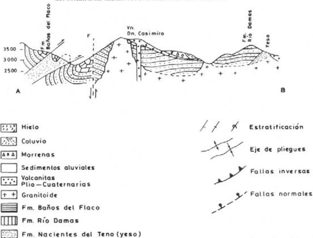
FIG. 2. Geología del área de los ríos Cruz de Piedra y Maipo superior y ubicación del volcán Don Casimiro. A: localidad de Las Tórtolas.
