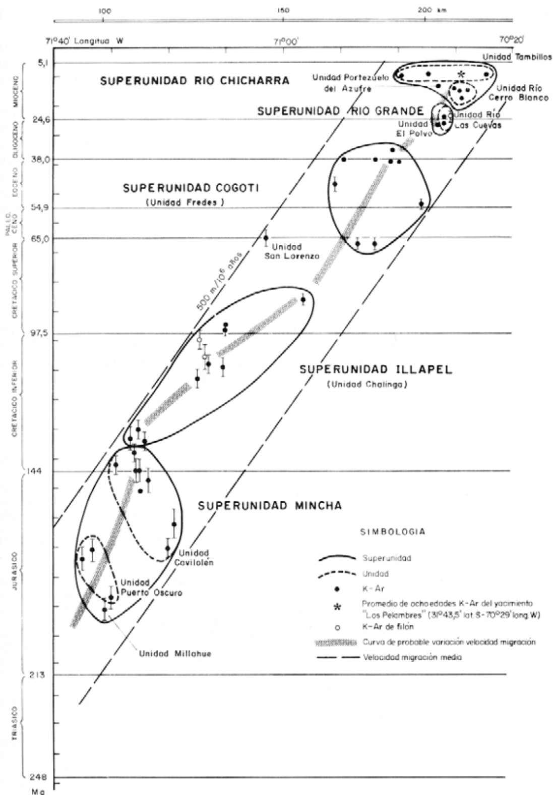
FIG. 2. Diagrama que relaciona edad versus longitud oeste y distancia a la posición de la fosa actual (Fuenzalida, 1983) de las rocas intrusivas mesocenoicas entre los 31° y 32° Lat. S.
