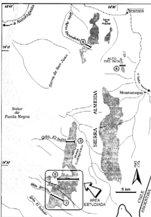
FIG. 8. Distribución de afloramientos de la Formación Zorritas en la Sierra Almeida. Los números indican los distintos lugares de control donde esta formación ha sido estudiada. 1- Quebrada del Agua Dulce; 2- Quebrada Zamolana; 3- Quebrada El Salto; 4- Quebrada Agua Escondida; 5- Alto del Inca.
