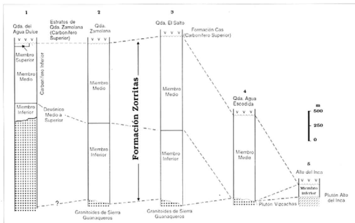
FIG. 9. Relaciones estratigráficas y espesores asignados a cada miembro de la Formación Zorritas según los principales lugares de control en Sierra Almeida, cuya ubicación aparece en figura 8. 1 y 2- esta contribución; 3- Isaacson et al. (1985); 4- Bahlburg et al. (1987); 5- Davidson et al. (1981).
