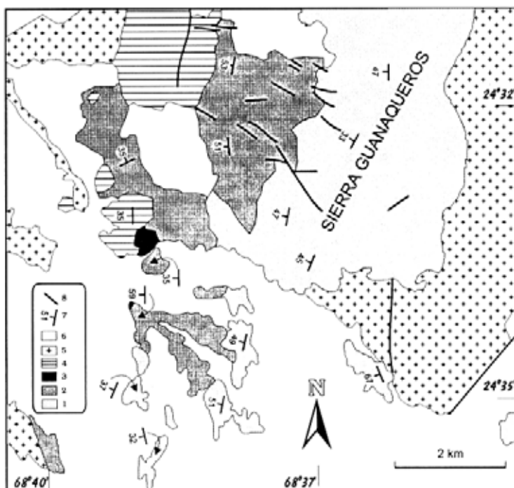
FIG. 2. Mapa geológico simplificado del área de la localidad tipo de la Formación Zorritas, mostrando la distribución de sus tres miembros. 1- Miembro Inferior (Devónico): cuarzoarenitas de grano fino a grueso, intercalaciones de conglomerados y limolitas; 2- Miembro Medio (Devónico-Carbonífero Inferior): limolitas, fangolitas y areniscas micáceas; 3- Miembro Superior (Carbonífero Inferior): areniscas de grano muy fino; 4- Estratos de Quebrada Zamolana (Carbonífero): riolitas, volcanoclastitas y sedimentitas; 5- granitoides de Sierra Guanaqueros (Paleozoico Superior): tonalitas y monzogranitos; 6- depósitos aluviales y volcanoclasticos aterrazados (Cenozoico Superior); 7- actitud de estratos; 8- fallas.
