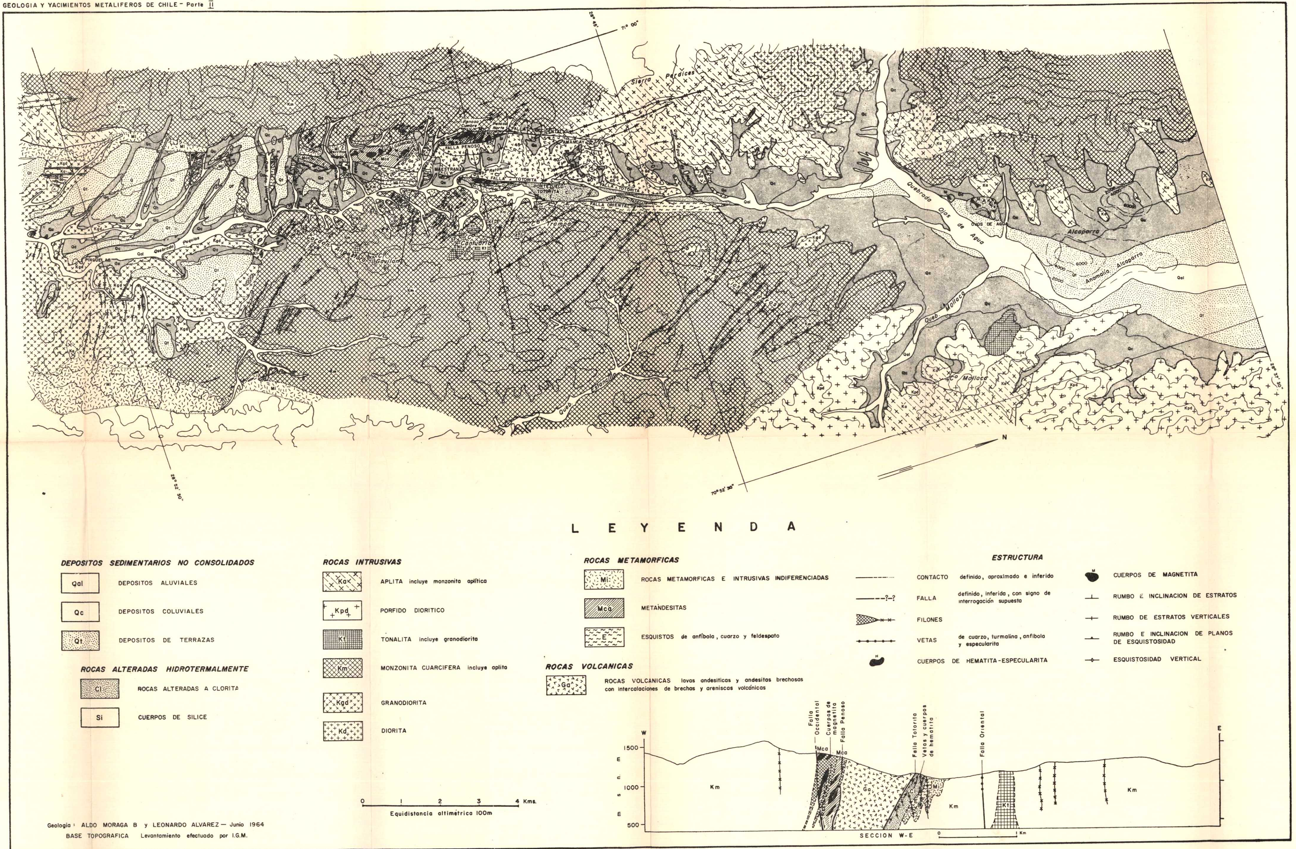
Figura 22. Geología del yacimiento de hierro El Algarrobo.
