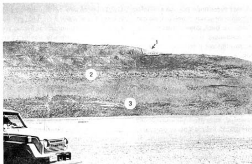
FIG. 7. Faldeo oriental, cerros de Soledad; se distinguen niveles de terrazas de borde, adosadas al cerro. Nótese nivel de acumulación, en terraza originalmente de abrasión (1).
