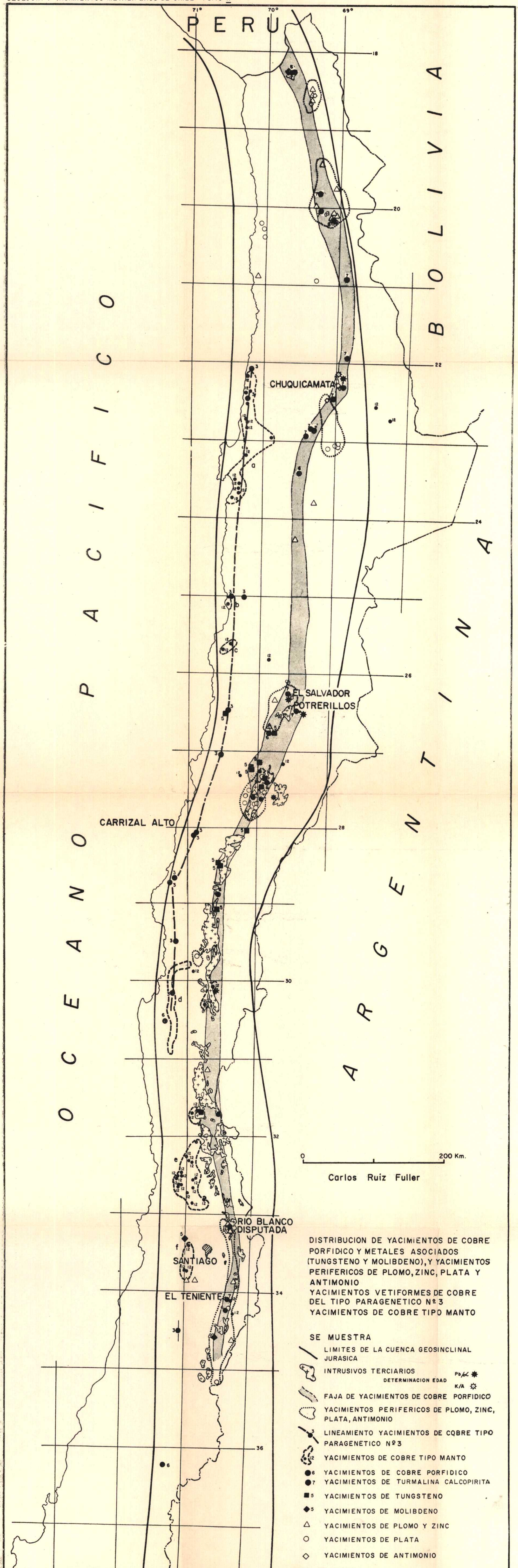
Figura I. Provincia Metalogénica del Geosinclinal Andino.
