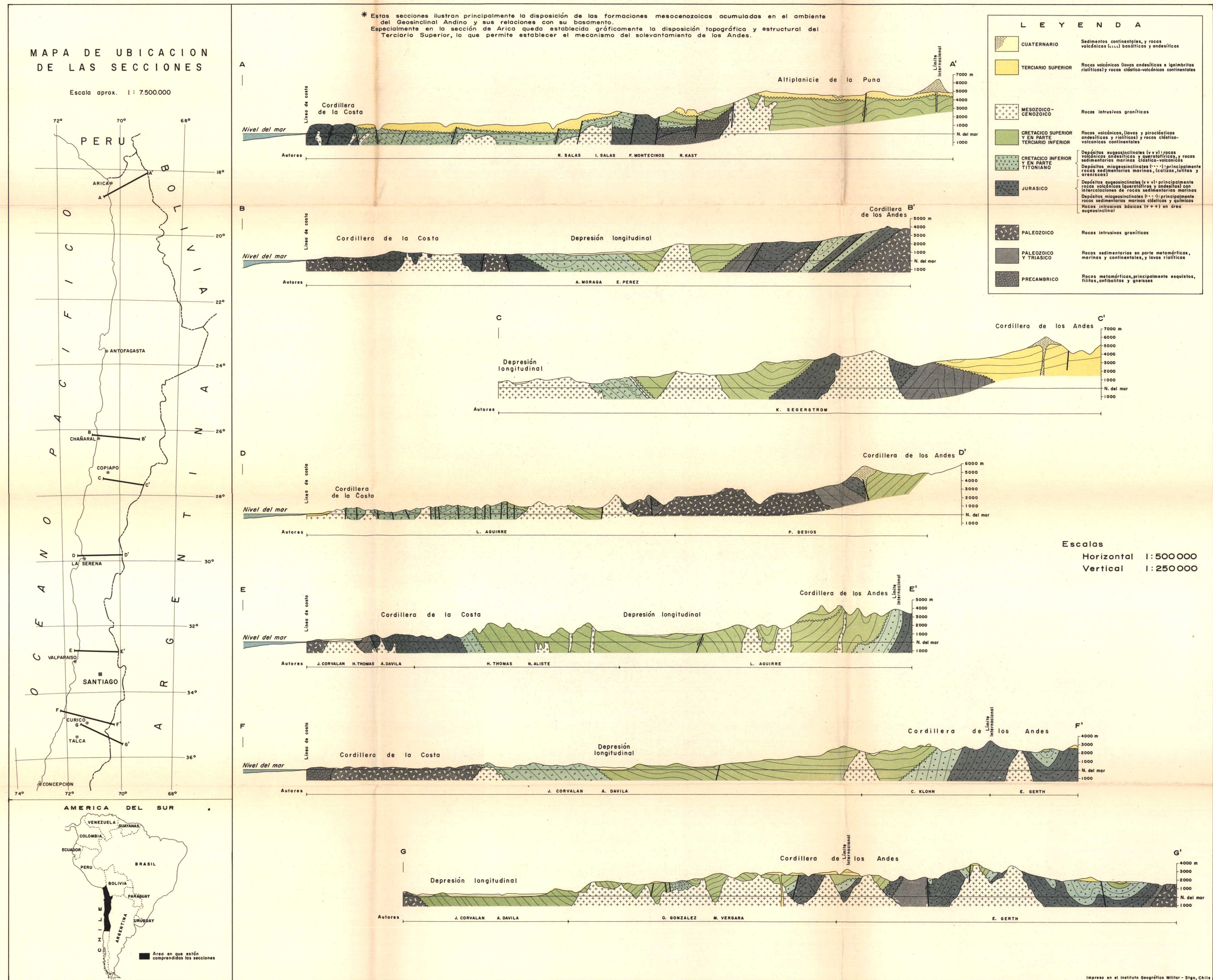
Figura II.- Secciones geológicas transversales del norte y centro de Chile.
